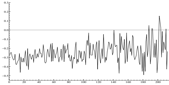
(d) MN2NGARCH skewness under Q
